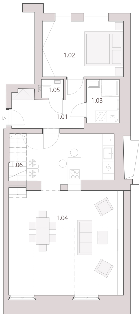
PŮDORYS 7.NP
